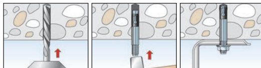
Kotwa gwoździowa FNA II A4 lub FNA II C z łbem płaskim - stal nierdzewna oraz stal o podwyższonej odporności na korozję 1.4529
